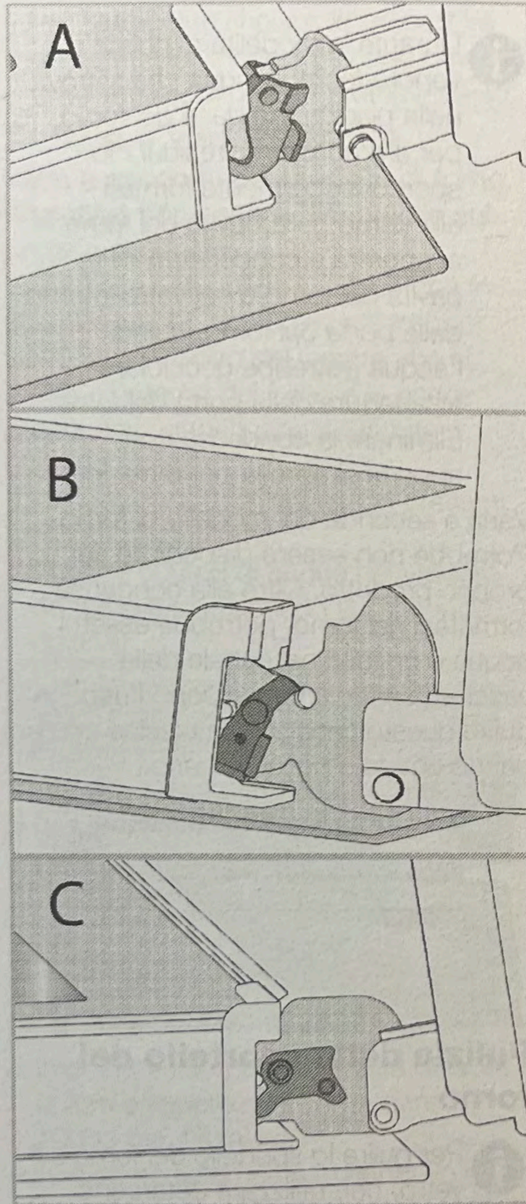
Serratura a cerniera - posizione aperta
